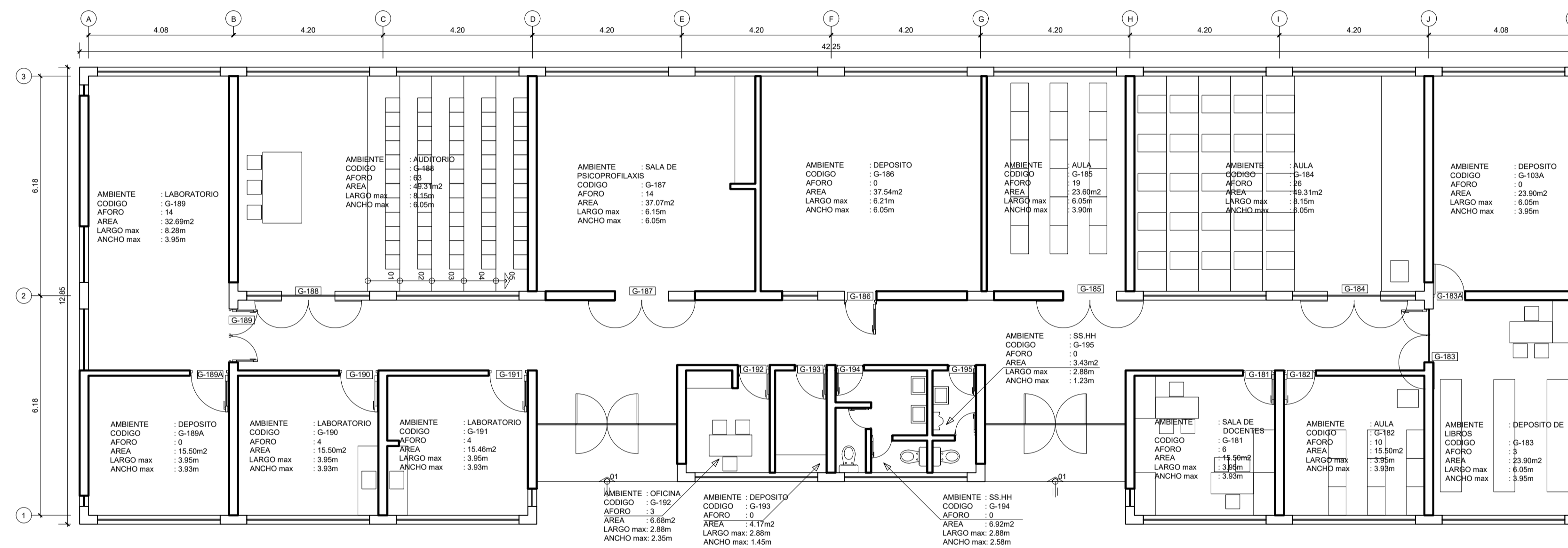
PRIMERA PLANTA AREA TECHADA = 523.05m 2 AFORO = 186 ESCALA 1:100
